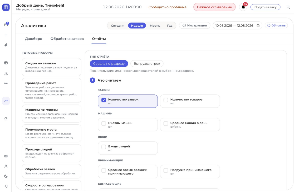
Рисунок 17.3 — Аналитика: отчёты
