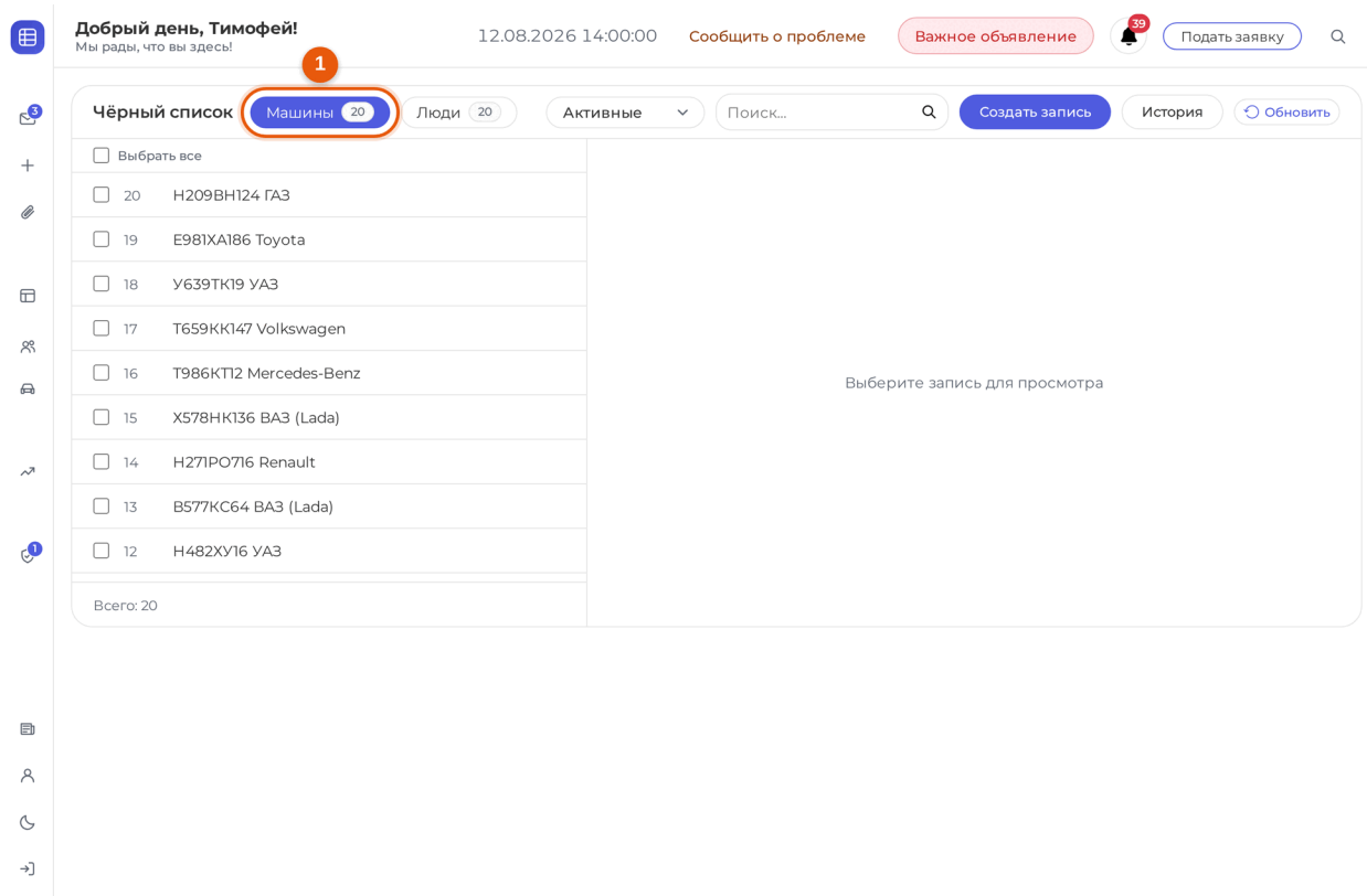
Рисунок 11.1 — Чёрный список
