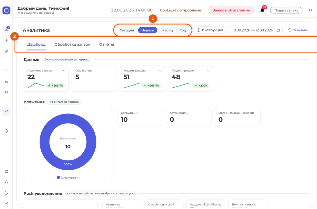
Рисунок 17.1 — Аналитика: дашборд
